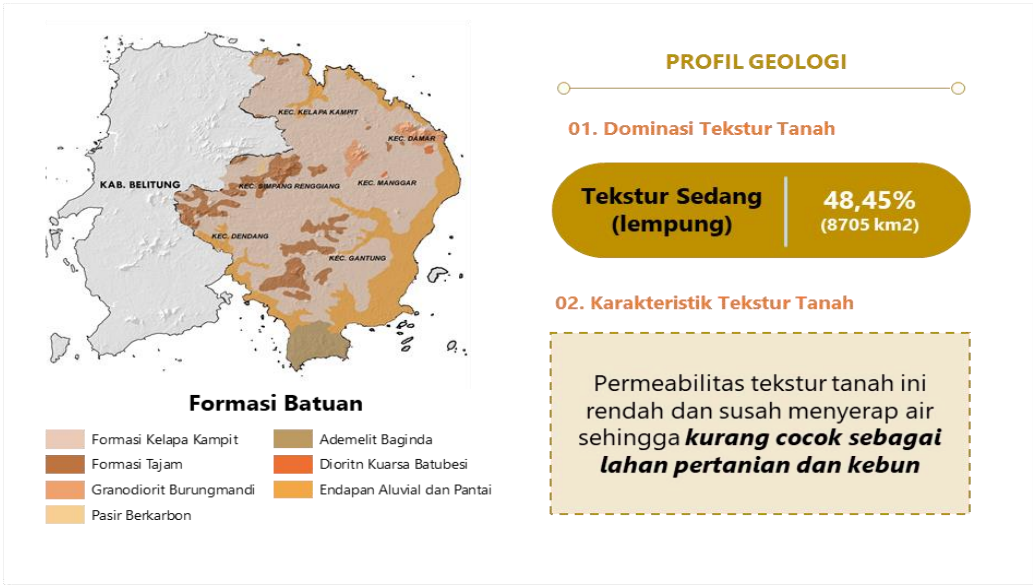
Gambar 2. 3 Kondisi Geologi Kabupaten Belitung Timur Sumber : Peta Geologi, Badan Geologi Kementerian ESDM tahun 2023
