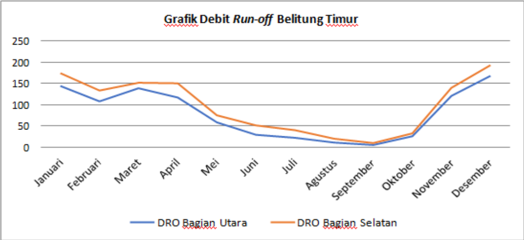
Grafik 2. 1 Debit Run-off Belitung Timur Tahun 2019 Sumber: Neraca Sumber Daya Alam Daerah Kab. Belitung Timur, 2019
